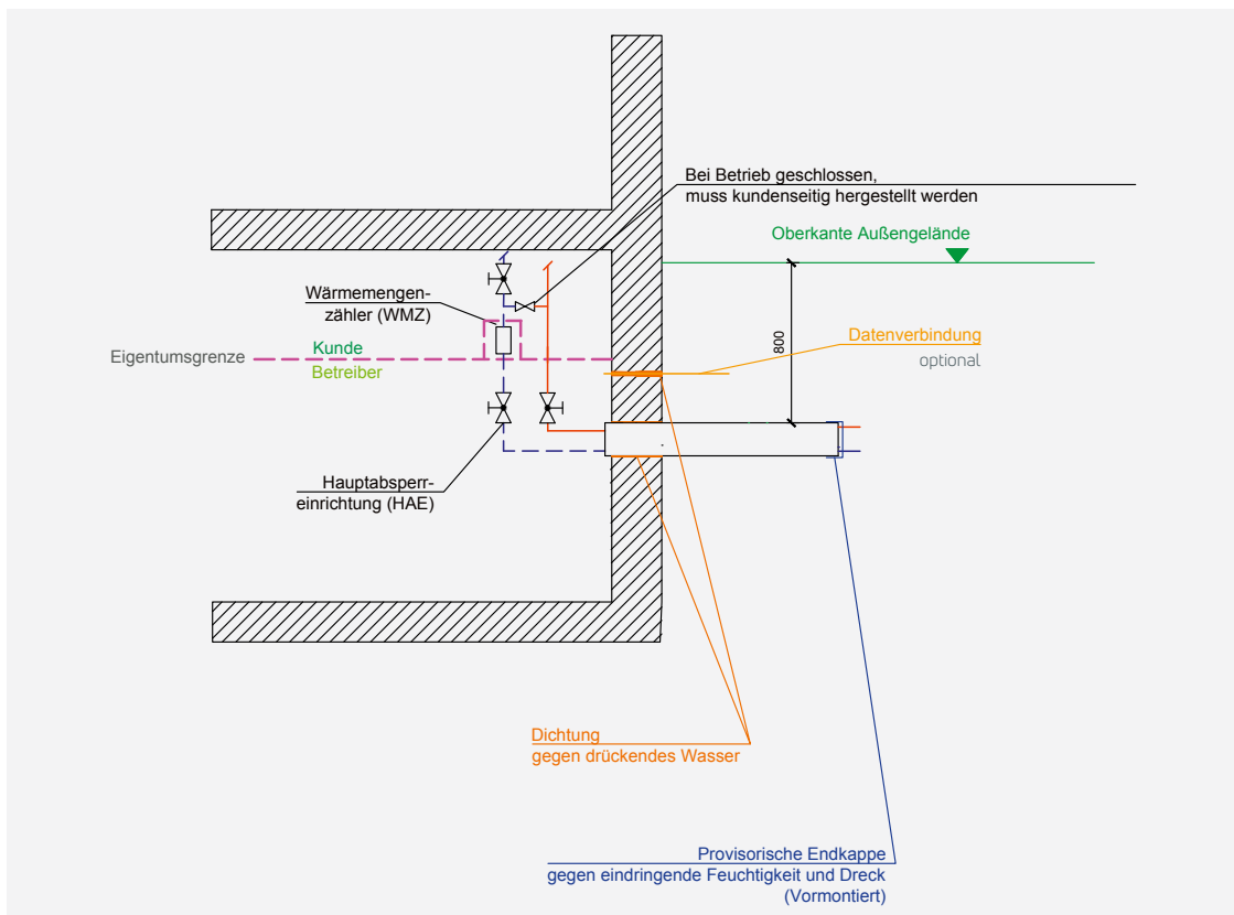
Abbildung 2: Hauseinführung Gebäude mit Keller
