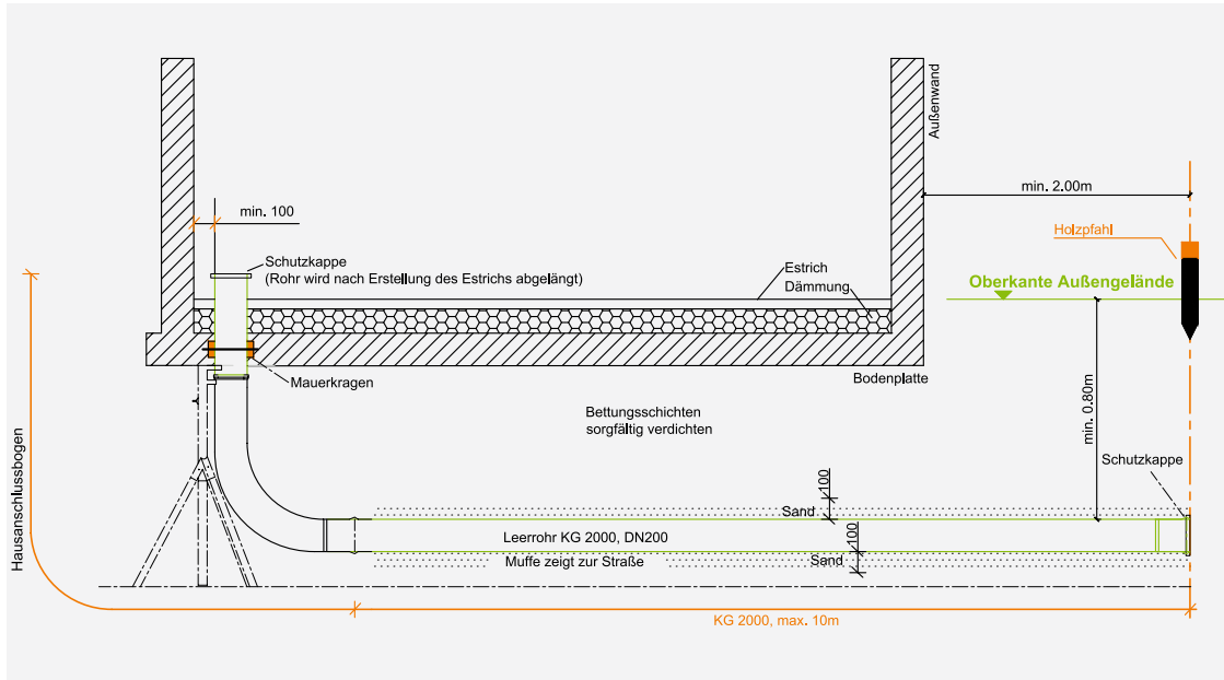
Abbildung 1: Hauseinführung Gebäude ohne Keller
