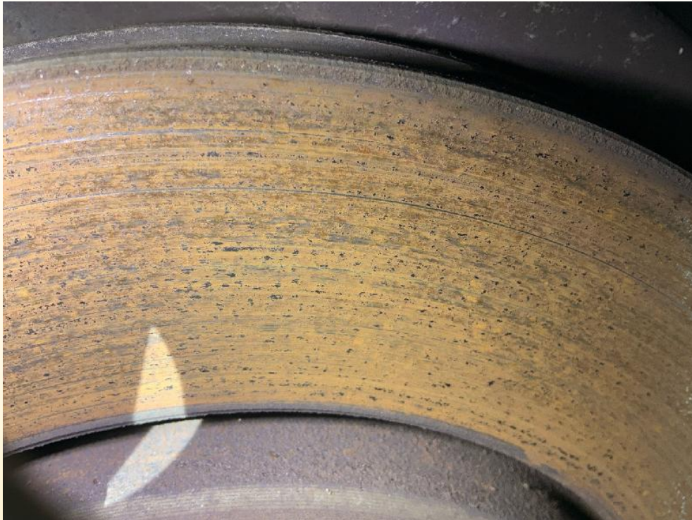
Bild: Betriebsbremse
