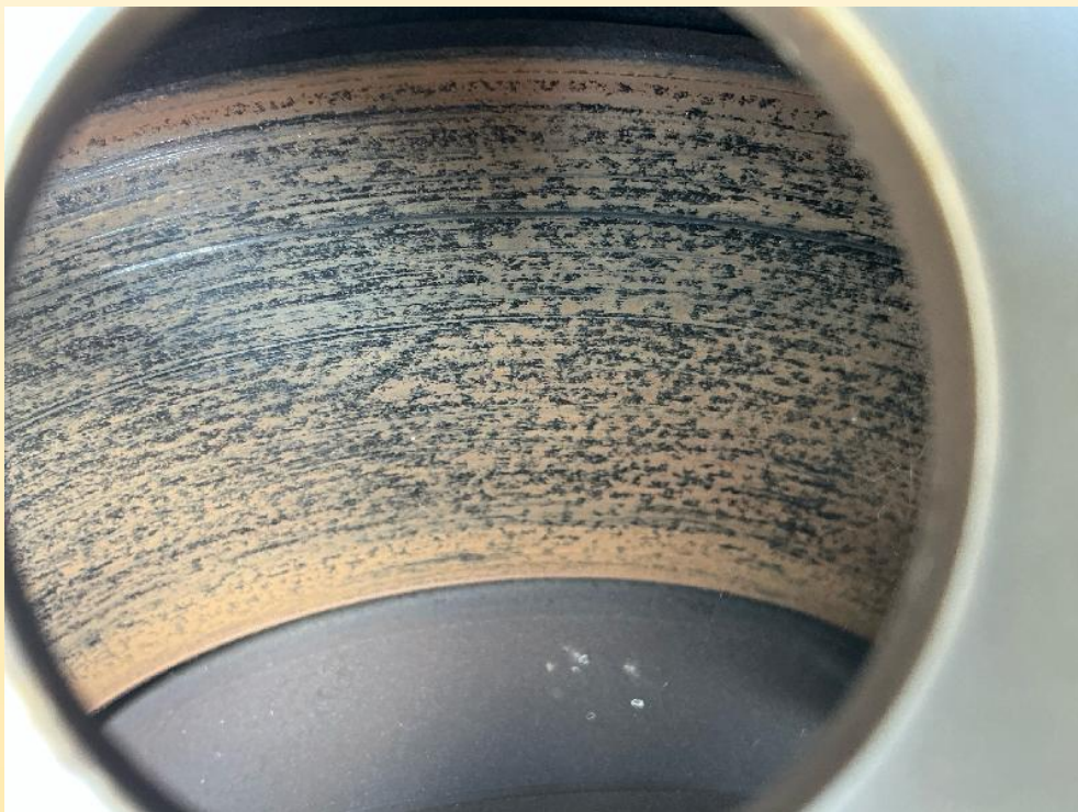
Bild: Betriebsbremse
